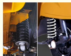
AMORTISSEURS AVANT ET ARRIÈRE TÉLESCOPIQUES ANTI-PLONGÉE
